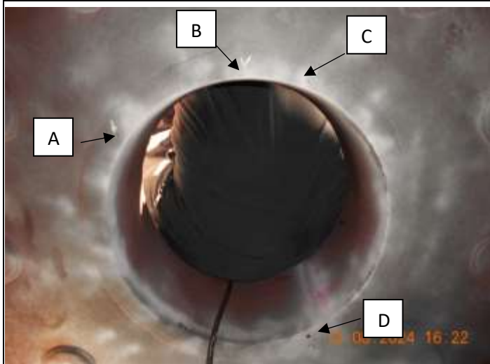
FOTO 3. Aplicacion de revelador se detectaron cuatro indicaciones.
